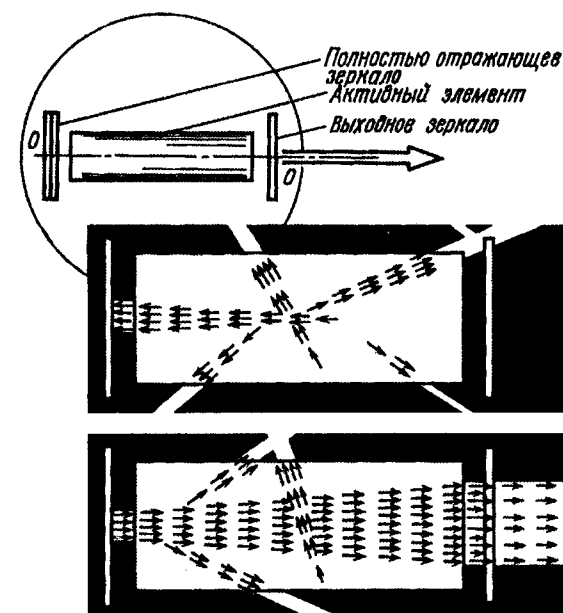
Рис. 1.10. Оптический резонатор выделяет в пространстве направление лазерной генерации (ось резонатора OO ) и создает наиболее благоприятные условия для развития процессов вынужденного испускания именно для данного направления
