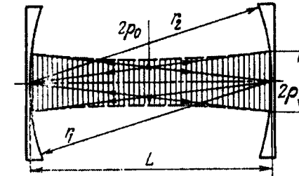
Рис. 2.29. Конфокальный резонатор (заштрихована область, занятая полем излучения внутри резонатора)
