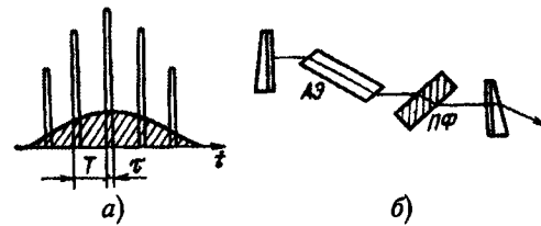
Рис. 3.8. Режим синхронизации продольных мод: а) гигантский импульс и последовательность сверхкоротких импульсов; б) резонатор, в котором предотвращена селекция продольных мод (АЭ — активный элемент; ПФ — просветляющийся фильтр, используемый при пассивной синхронизации мод)
