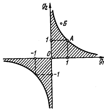
Рис. 2.28. Диаграмма устойчивости резонаторов
