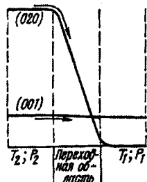
Рис. 2.21. Характер изменения заселенностей верхнего и нижнего рабочих уровней молекулы \text{CO}_2 по мере перехода газовой смеси из форкамеры в объем резонатора
