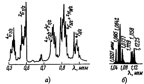
Рис. 2.7. Спектры поглощения иона неодима (а) и люминесценции неодима (б) в гранате (спектр люминесценции дан для переходов 4F_{3/2} \rightarrow 4I_{11/2} )
