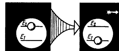
Рис. 1.7. Спонтанное испускание света
