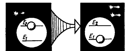
Рис. 1.6. Вынужденное испускание света
