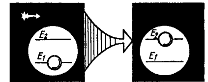
Рис. 1.5. Поглощение света
