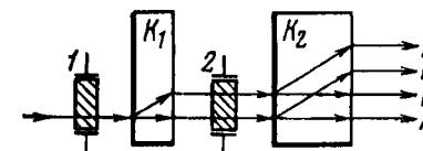
Рис. 3.17. Электрооптический дефлектор дискретного действия (двухкаскадная схема)
