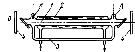
Рис. 2.15. Аргоновый лазер: А — анод; К — катод; 1 — рабочий объем газоразрядной трубки; 2 — система водяного охлаждения; 3 — обводной канал; 4 — зеркала оптического резонатора
