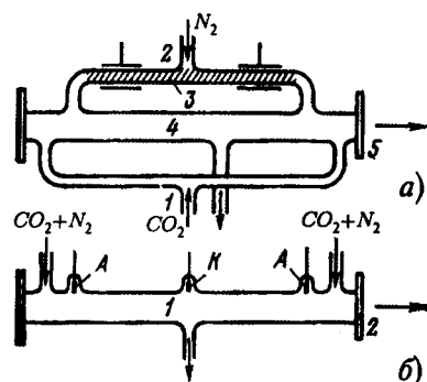
Рис. 2.17. Два варианта CO 2 -лазера: а) с разделением областей разряда и рабочего объема резонатора (1 — система прокачки двуокиси углерода, 2 — система прокачки азота, 3 — область высокочастотного тлеющего разряда, 4 — рабочий объем резонатора, 5 — выходное зеркало резонатора); б) с совмещением областей разряда и рабочего объема резонатора (А — анод, К — катод, 1 — рабочий объем резонатора, 2 — выходное зеркало резонатора)
