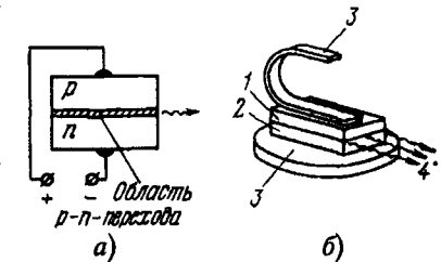
Рис. 2.26. Инжекционный лазер: а) принципиальная схема лазера; б) внешний вид лазера (1 — p -полупроводник; 2 — n -полупроводник; 3 — металические контакты; 4 — излучение лазера)
