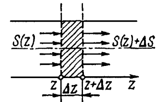
Рис. 1.14. Усиление светового потока в тонком слое инвертированной активной среды
