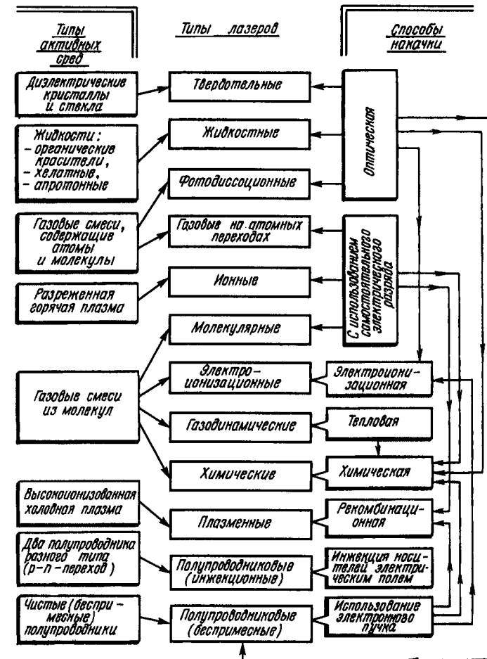
Рис. 2.1. Классификация лазеров
