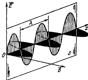
Рис. 1.1. Схематическое изображение электромагнитной волны. Волна является плоской, идеально монохроматической, идеально поляризованной. Плоский волновой фронт ориентирован перпендикулярно к направлению распространения волны (перпендикулярно к оси z )
