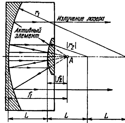
Рис. 2.30. Неустойчивый резонатор телескопического типа: f_1 и f_2 — фокусные расстояния зеркал; точка A — общий фокус зеркал
