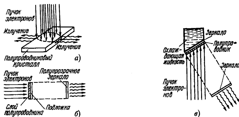
Рис. 2.24. Схемы полупроводниковых лазеров, возбуждаемых электронным пучком: а) с поперечной накачкой; б) с продольной накачкой (1-й вариант); в) с продольной накачкой (2-й вариант)
