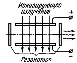
Рис. 2.10. Схема, поясняющая электроионизационную накачку
